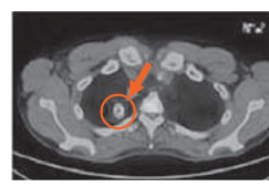
PET-CT画像
