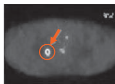
PET画像
